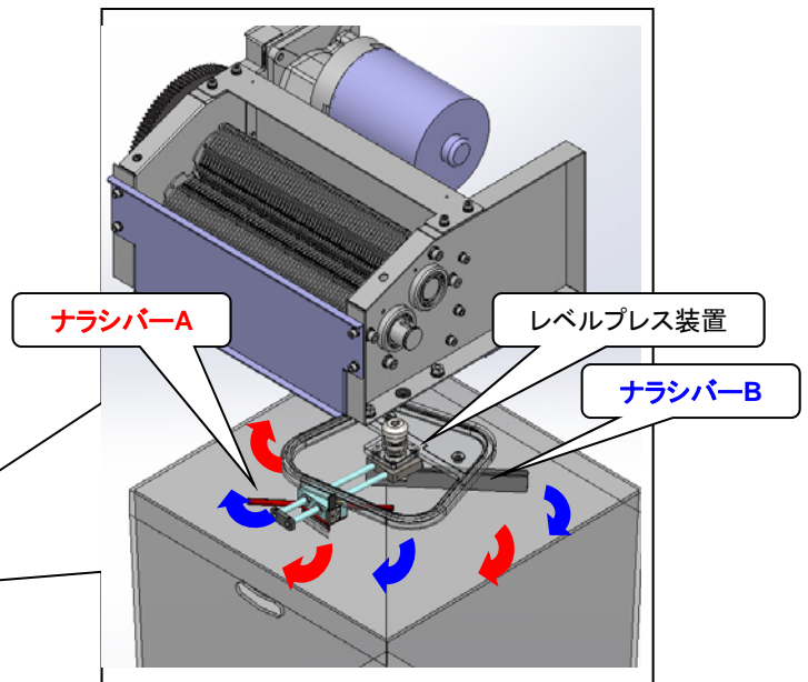
ナラシパーA・Bの軌道(上面図)
